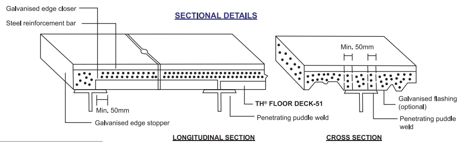
LONGITUDINAL SECTION
