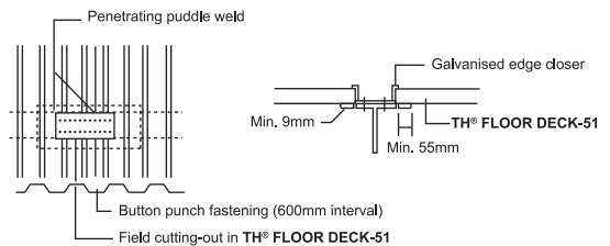
LONGITUDINAL SECTION
