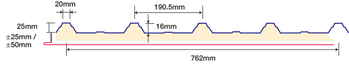
PU Foam Metal
